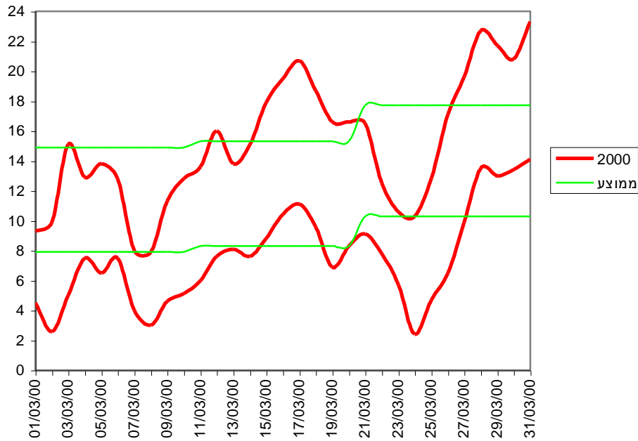
מפרטורת מינימום ומקסימום יומית בירושלים במרס 0002 יחסית לממוצע
