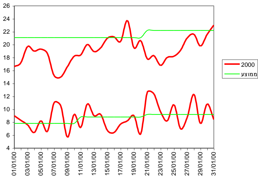
מפרטורת מינימום ומקסימום יומית בבית דגן במרס 0002 יחסית לממוצע
