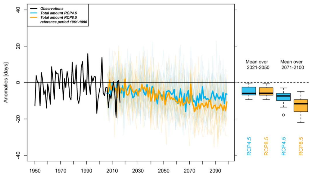
איור 12. כמו איור 11 רק עבור מספר ימי הגשם (יום גשם מוגדר להיות 1 מ"מ/יום ומעלה).
