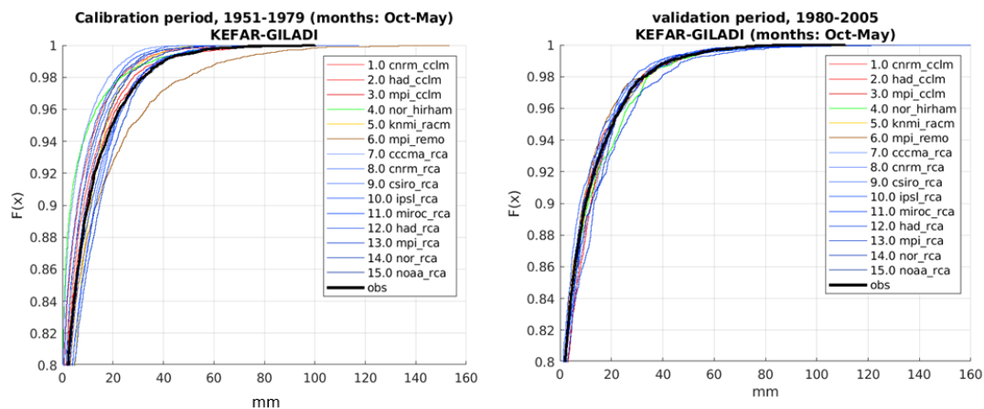
איור 19. דוגמה מתחנת כפר גלעדי, לתיקון המודלים השונים באמצעות QDM, עבור כמויות הגשם, בתקופת האימות. בפאנל השמאלי ניתן לראות את התפלגות התצפיות בשחור ואת האופן בו המודלים השונים (בגווני צבעוניים) דימו את כמויות הגשם בתקופה 1979-1951. בפאנל הימני מוצגת התפלגות התצפיות מול התפלגויות המודלים השונים לאחר תיקון, בתקופת האימות 2005-1980. התפלגויות המודלים לאחר התיקון הרבה יותר דומות למדידות שהיו בתחנה (הדבר גם נתמך אמפירית באמצעות שימוש ב-Kolmogorov-Smirnov test).
