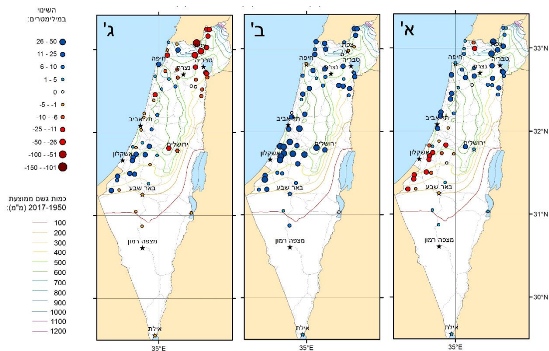
איור 14. השינוי בכמות המשקעים השנתית הממוצעת (מ"מ) ביחס לתקופה 1951-2017 בתקופות: א) 1951-1980, ב) 1971-2000, ג) 2000-2017.
