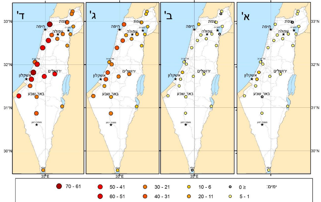
איור 6. השינוי במספר הימים בהם טמפרטורת המקסימום גדולה מ-30°C בממוצע ביחס לתקופה 1990-1961 בתקופות: א) 1979-1950, ב) 2000-1971, ג) 2017-1988, ד) 2050-2021 לפי תרחיש RCP8.5.
