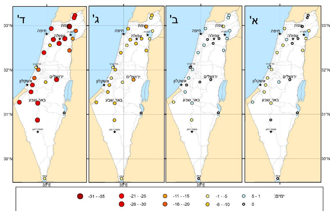
איור 4. השינוי במספר הימים בהם טמפרטורת המינימום קטנה מ-7 מ"צ בממוצע ביחס לתקופה 1990-1961 (בתקופות: א) 1979-1950, ב) 2000-1971, ג) 2017-1988, ד) 2050-2021 לפי תרחיש RCP8.5.
